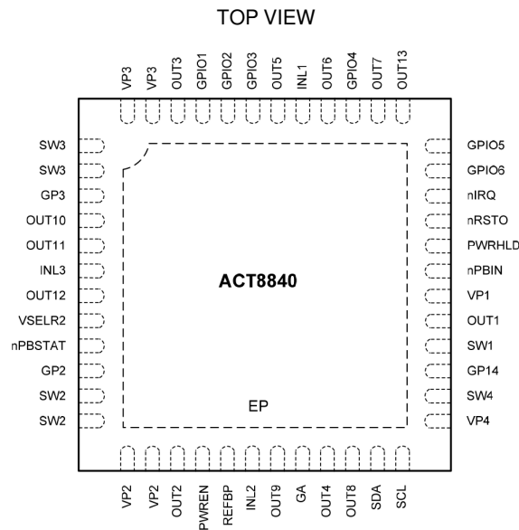
Thin - QFN (TQFN66-48)
