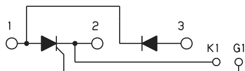
回路構成 Circuit Schema
