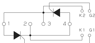
回路構成 Circuit Schema
