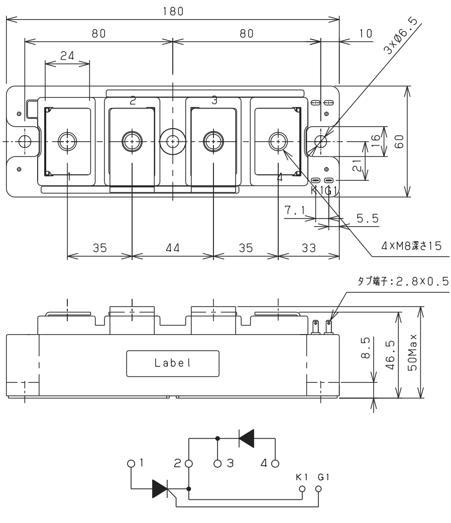
回路構成 Circuit Schema
