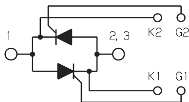
回路構成 Circuit Schema
